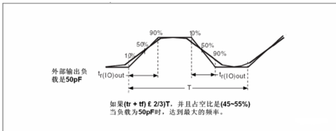
图15. 输入输出交流特性定义
