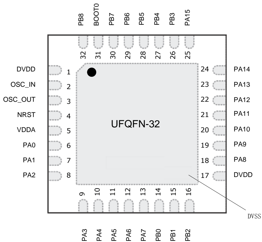
图5. MM32F031UFQFN32引脚分布
