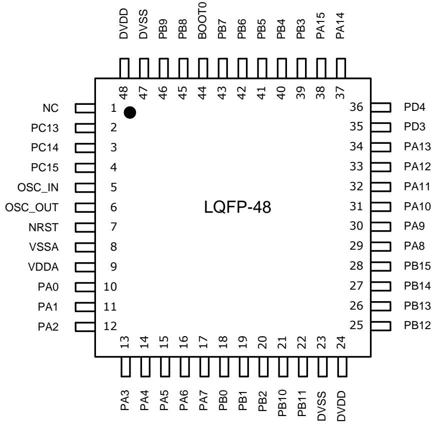
图3. MM32F031LQFP48引脚分布
