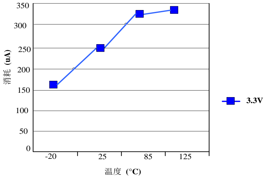
图12. 待机模式下的典型电流消耗在 V_{DD}=3.3V （和 3.6V ）时与温度的对比
