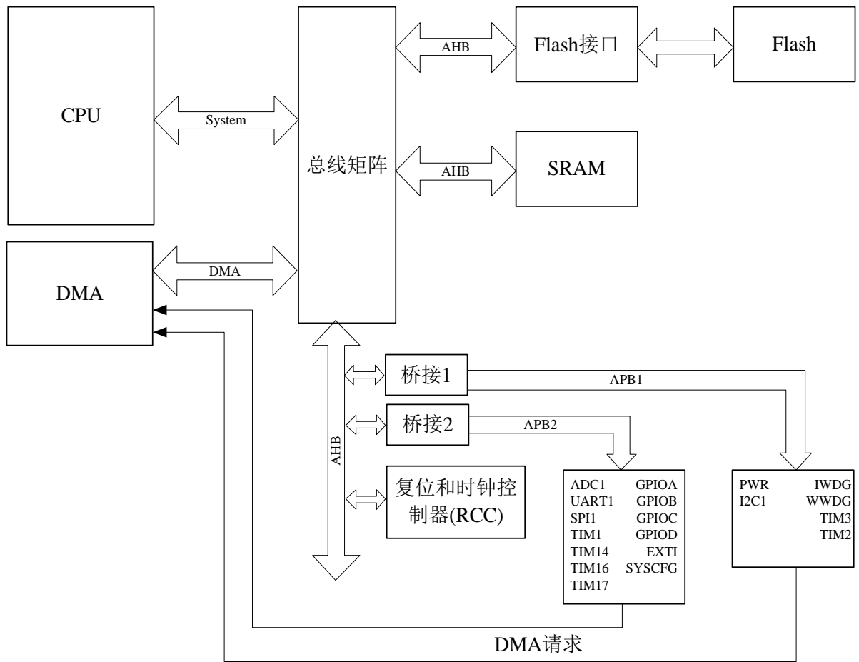
图1. MM32F031模块框图
