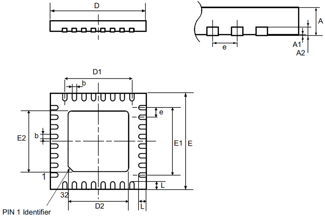
图26. UFQFN-32, 方形扁平无引线封装外形
