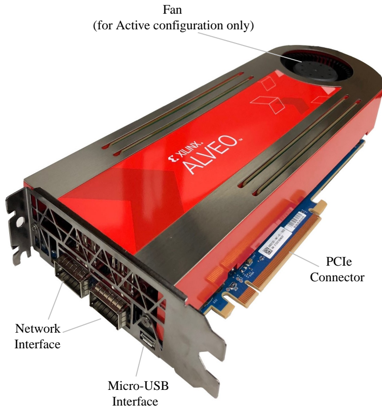
图 1: U200/U250 卡功能
