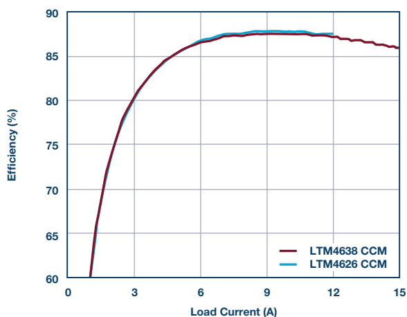
图 5. LTM4626 和 LTM4638 的效率 (12 V 输入、1 V 输出、600 kHz 工作频率)。
