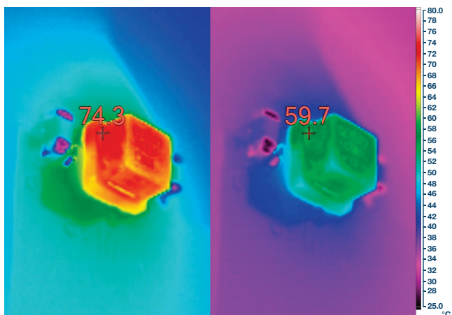
图 4. 在该对比中 (0 LFM 和 200 LFM 气流), CoP 设计的有效气流冷却对 LTM4638 热性能的影响清晰可见 (12 V 输入、1 V/15 A 输出)。
