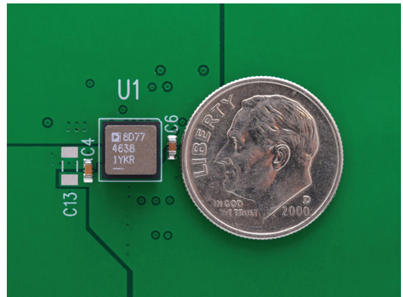
图 2. 纤巧型 15 A DC/DC \mu Module 稳压器解决方案 (采用了安装在一块 DC2665A-B 演示板上的 LTM4638)。这里示出了输入和输出电容——少量的陶瓷电容和一个电路板背面的电阻。
