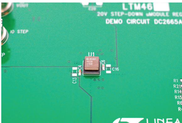
图 6. DC2665A-A 演示板上的 LTM4626。
