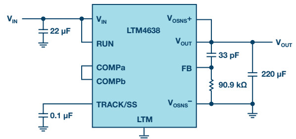
图 3. LTM4638 12 V 输入、1 V 输出、600 kHz 简化原理图 (仅采用陶瓷电容和极少的组件)。图中未示出浮置引脚。
