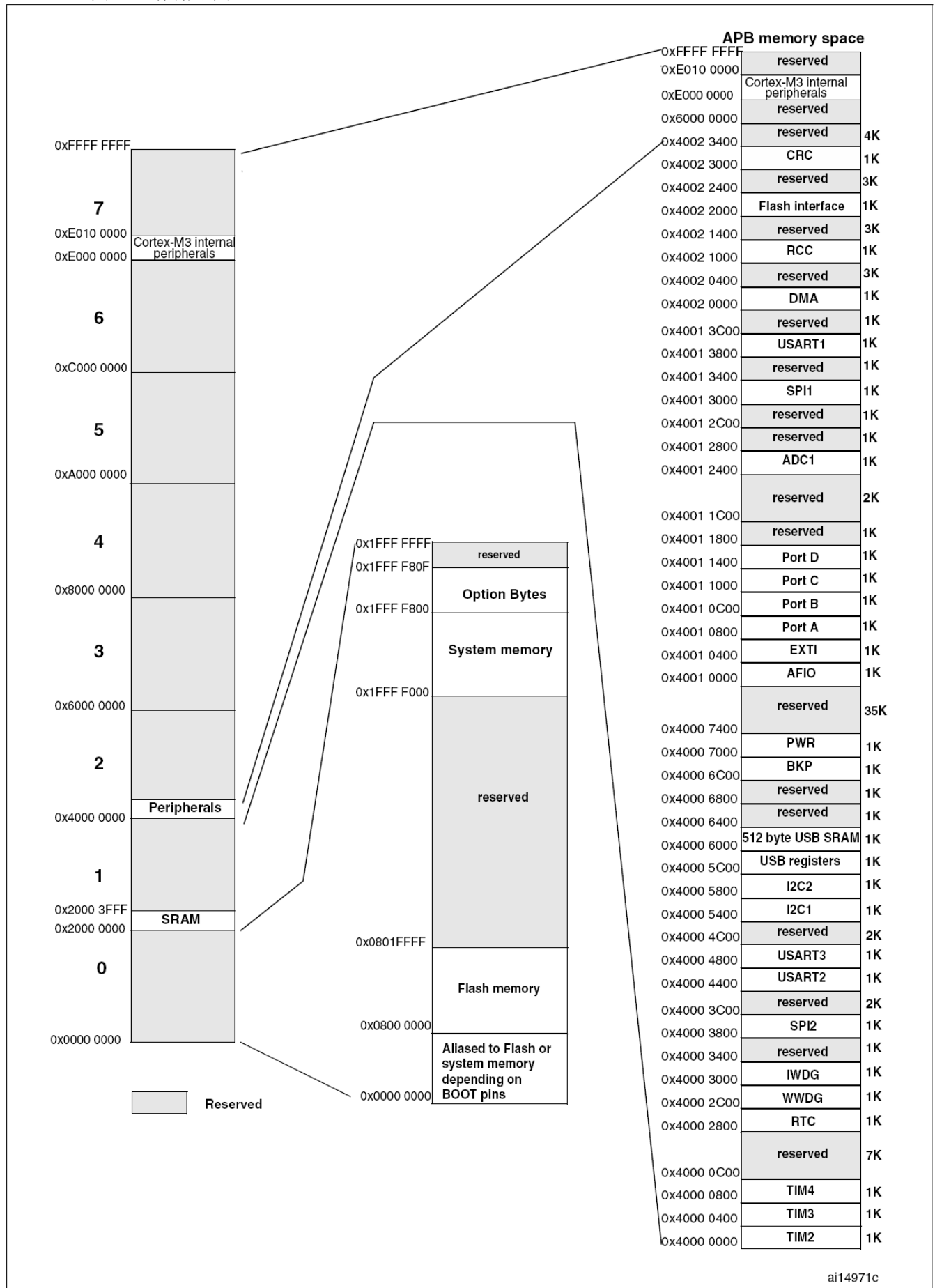
图5 存储器图
