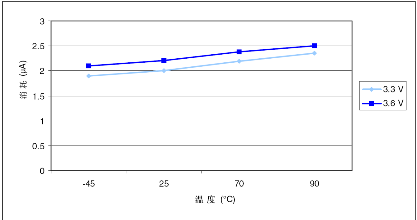
图15 待机模式下的典型电流消耗在 V_{DD}=3.3V 和 3.6V 时与温度的对比
