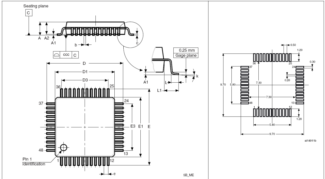
图33 建议的PCB元件尺寸 (1)(2)
