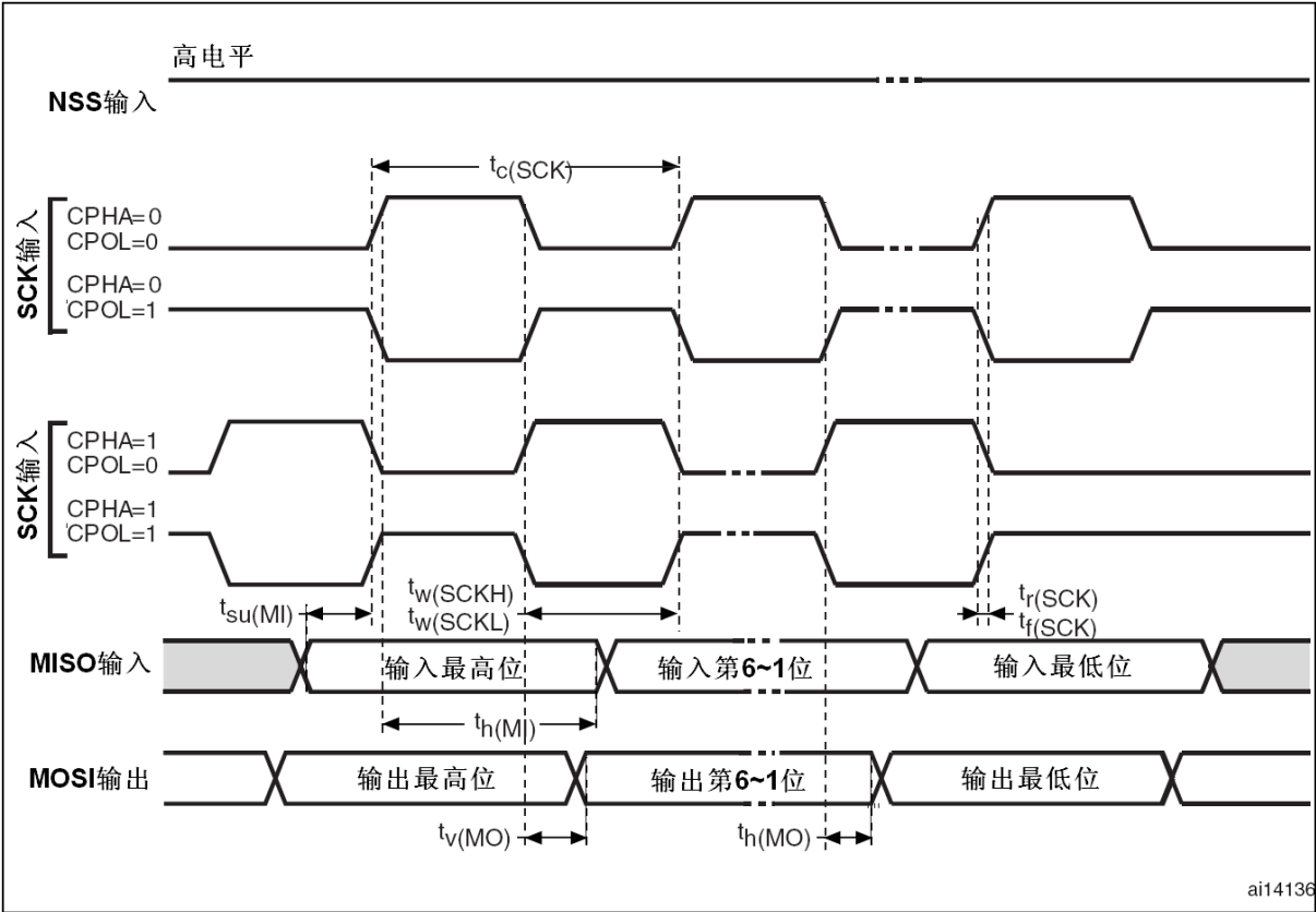
图25 SPI时序图 – 主模式 (1)
