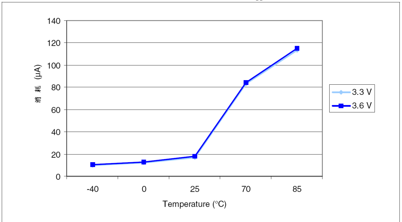
图14 调压器在低功耗状态时，停机模式下的典型电流消耗在 V_{DD}=3.3V 和 3.6V 时与温度的对比
