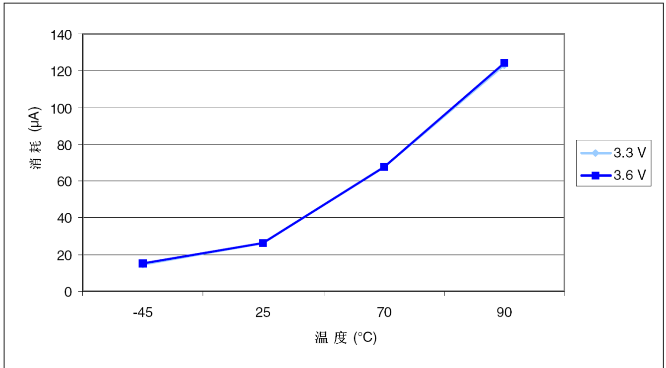
图13 在调压器在运行状态时，停机模式下的典型电流消耗在 V_{DD}=3.3V 和 3.6V 时与温度的对比
