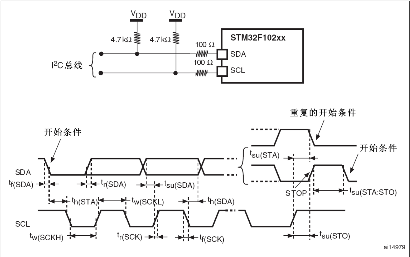
图22 I 2 C总线交流波形和测量电路 (1)
