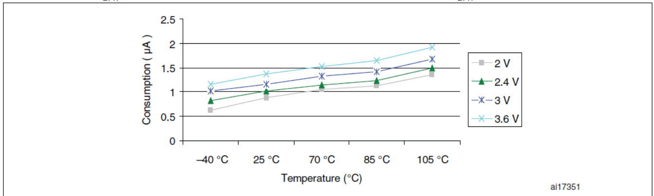
图12 由 V_{BAT} 供电, 并使能RTC功能的情况下, 典型功耗电流在不同 V_{BAT} 供电时随温度的变化图
