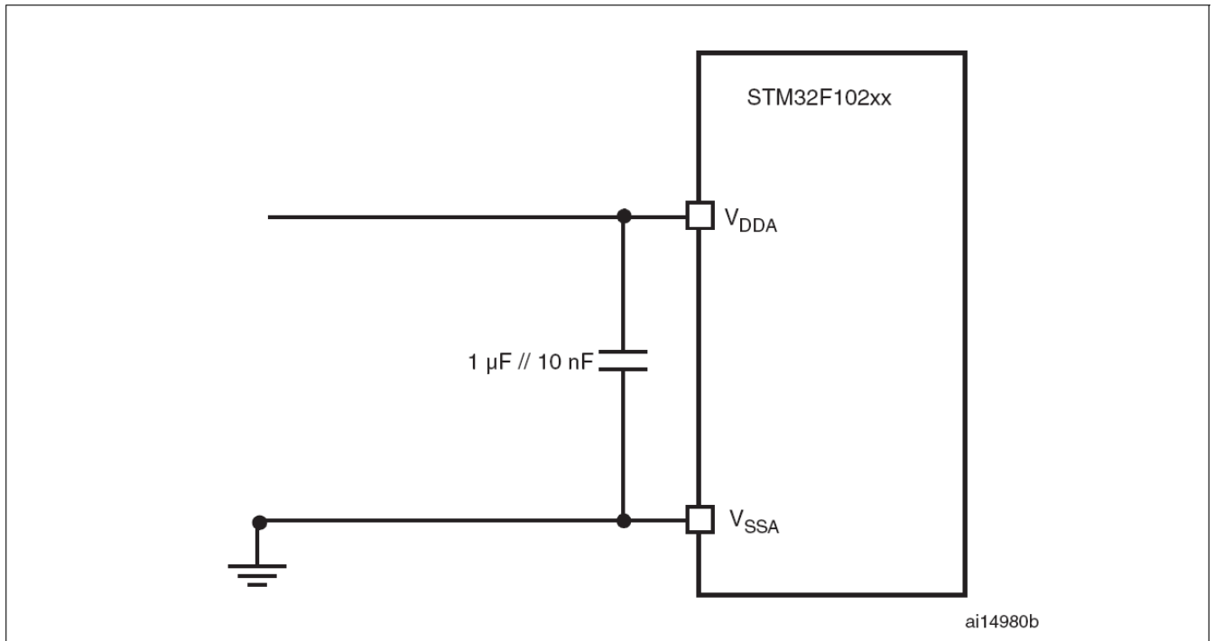
图29 供电电源和参考电源去耦线路
