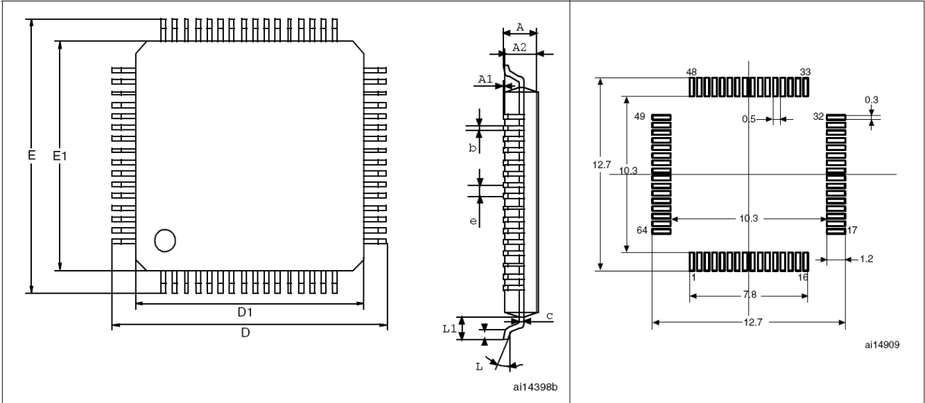
图31 建议的PCB图(尺寸以mm为单位) (1)
