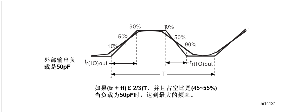
图20 输入输出交流特性定义
