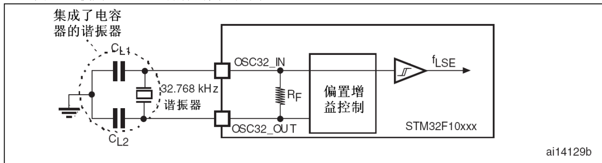
图19 使用32.768kHz晶体的典型应用
