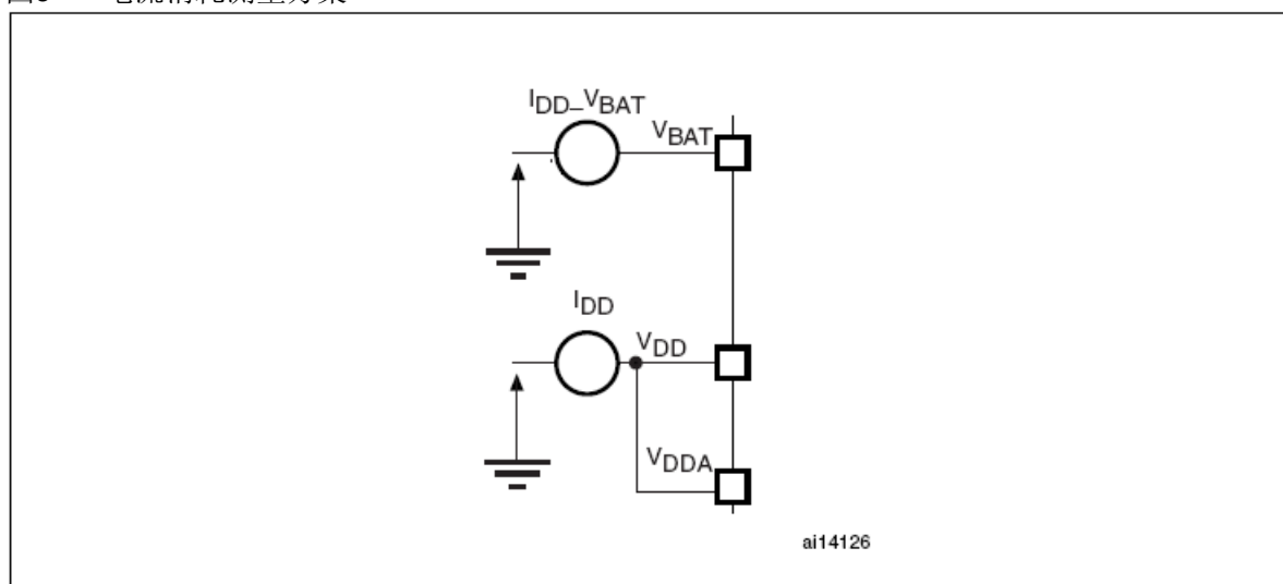
图9 电流消耗测量方案
