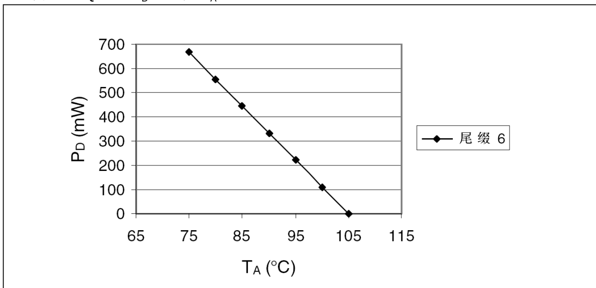
图34 LQFP64 P_{Dmax} 对照 T_A
