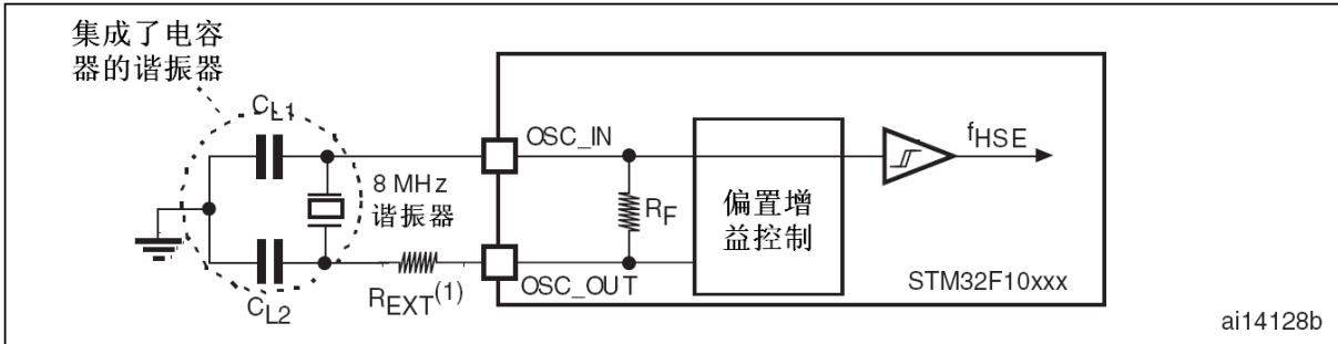
图18 使用8MHz晶体的典型应用
