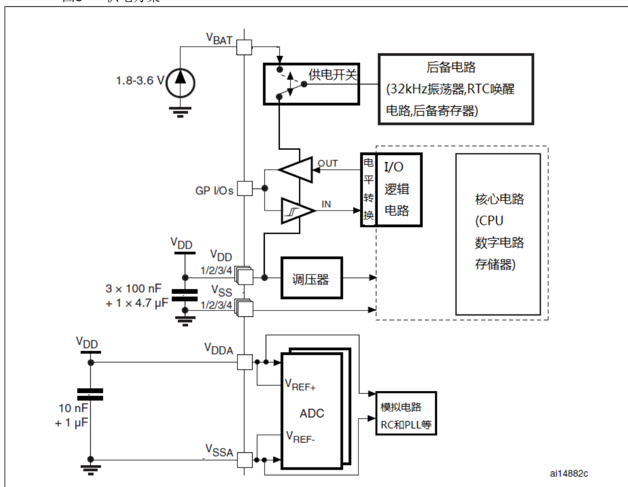
图8 供电方案
