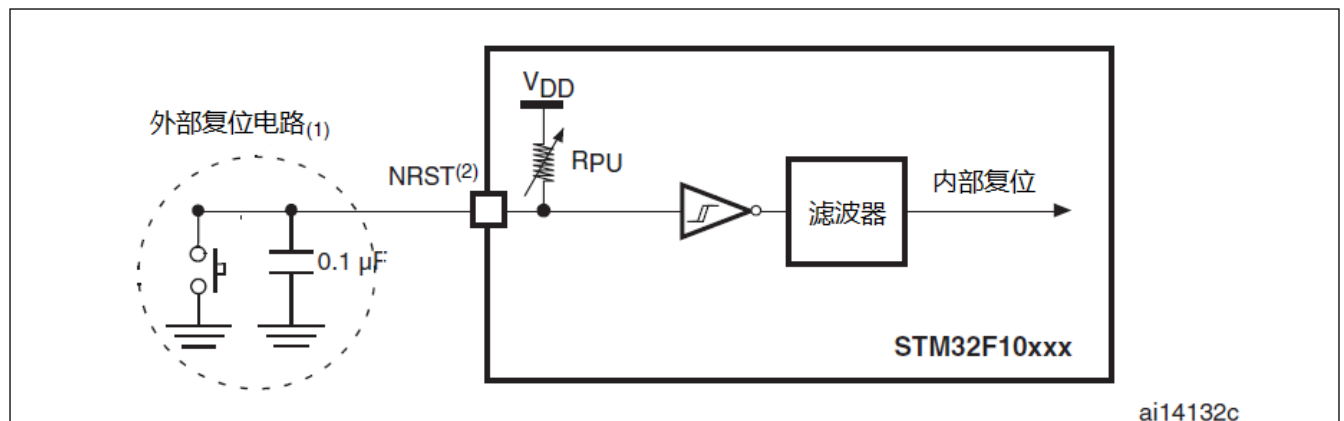
图21 建议的NRST引脚保护
