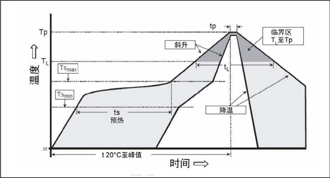
图3. 推荐的回流焊曲线
