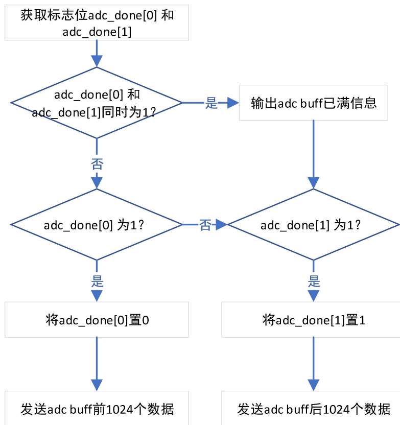
图 4-1 LWIP TCP 发送 ADC 数据流程
