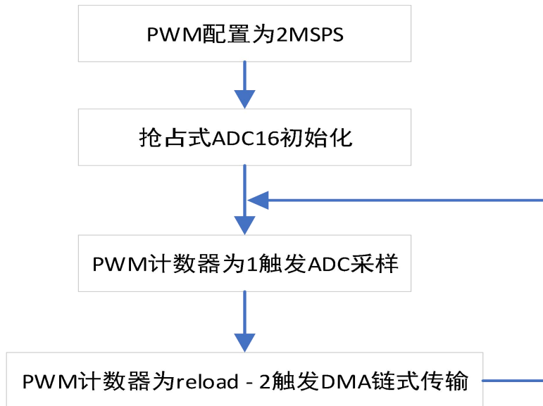
图 3-1 PWM 触发 ADC16 采样 流程
