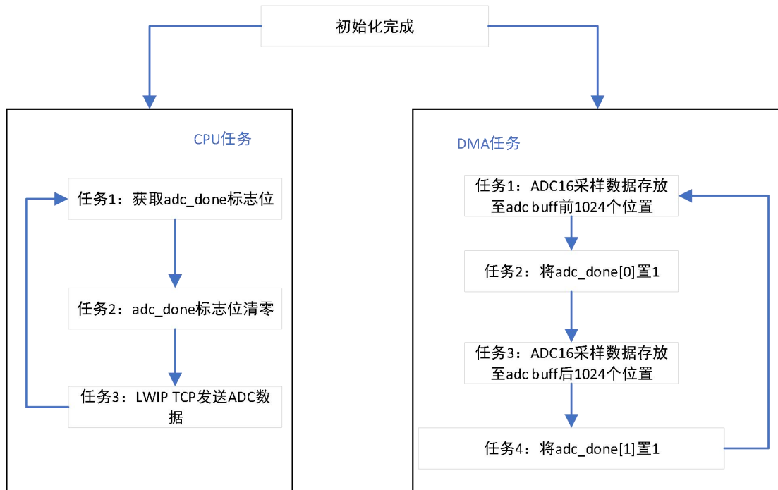
图 2-2 CPU 任务与 DMA 任务并行运行
