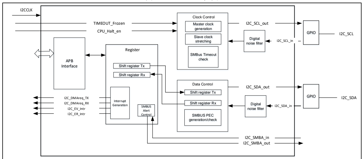
图 2. I 2 C2、I 2 C3 框图
