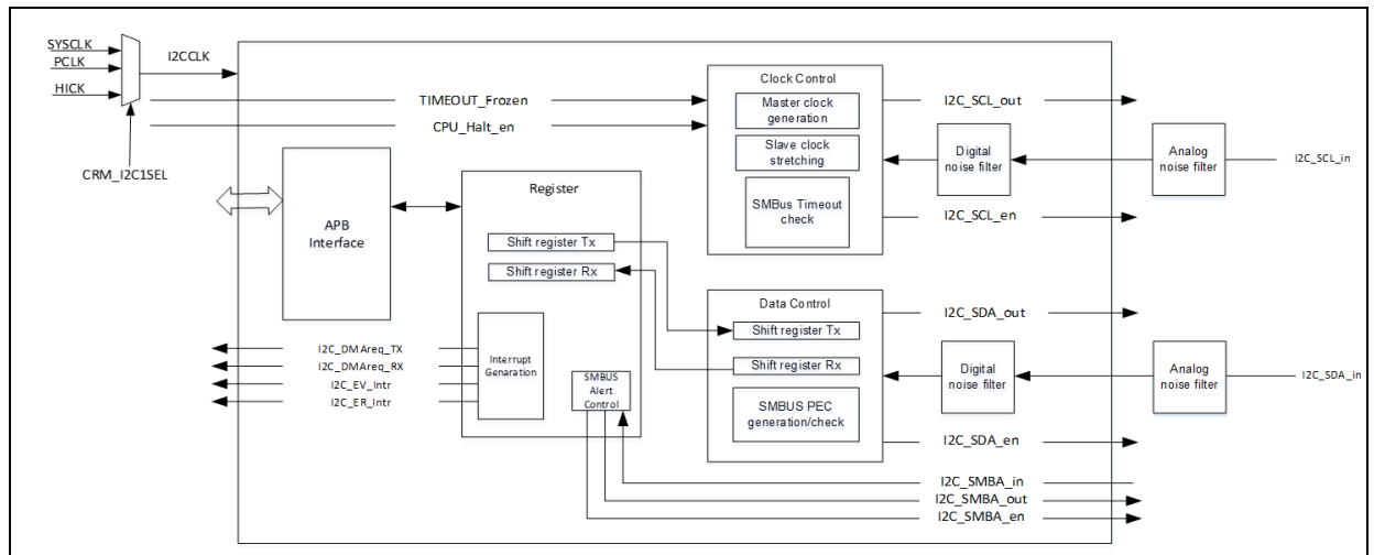
图 1. I 2 C1 框图
