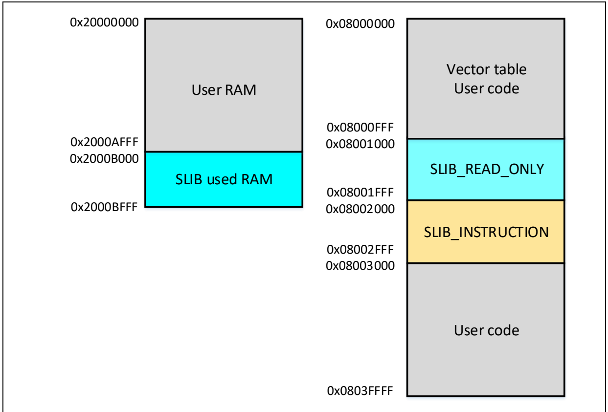
图 13. 范例程序的主闪存映像及 RAM 分区
