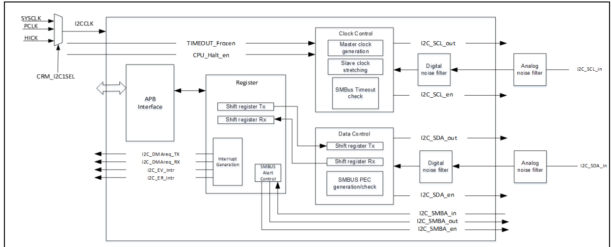
图 1. I 2 C 框图
